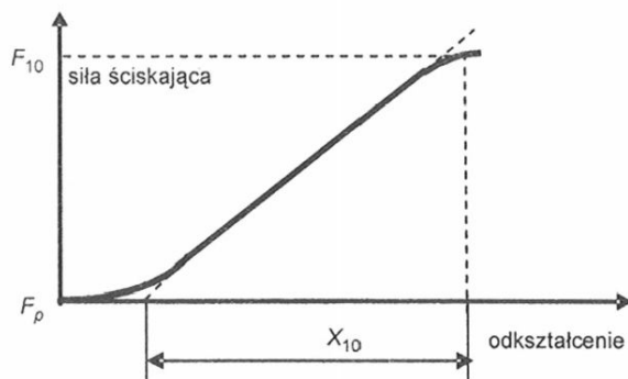
Rys. 1. Przykład zależności siły od odkształcenia Fig. 1. Example relationship between force and deformation
